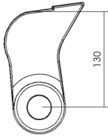
Figura 7.4 Limite de desgaste de las cuchillas
