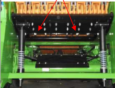
Rastrillo Tuerca
