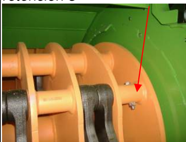
Figura 7.6 Retirar los tornillos de retención 3
